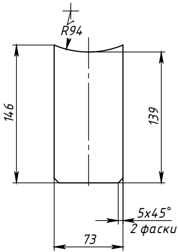
Поз.3 (Ребро)
