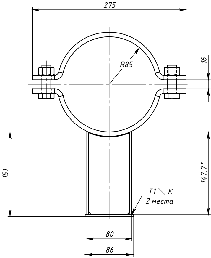
Поз.4 (Полухомут)
