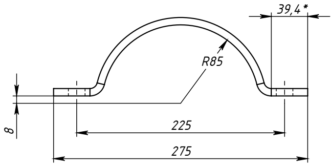
Поз.4 (Полухомут)
